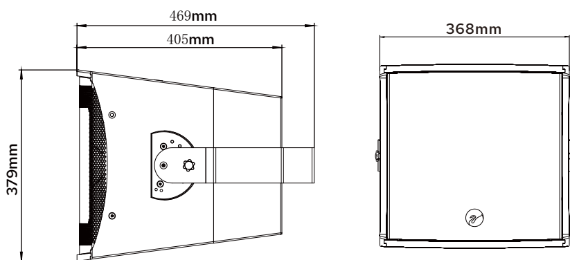
产品外尺寸
