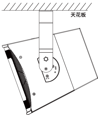
天花吊挂
