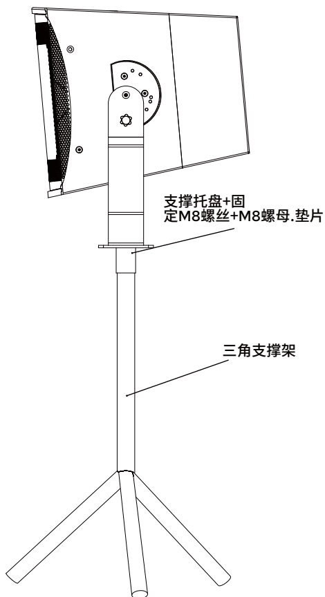
三脚架支撑
