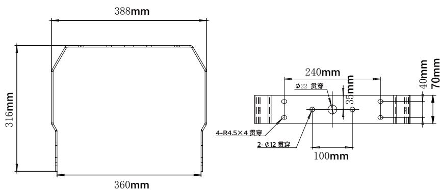
挂架尺寸
